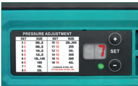
Bedienelement zur Druckparameter-Einstellung (Vorgaben auf der Maschine angegeben) inkl. Statusleuchten
