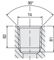
Einschraubloch (Kegeliges Gewinde)
