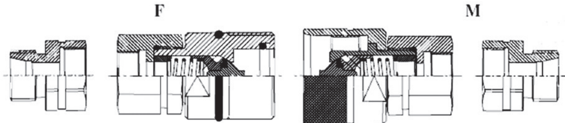
Serie " 30 " 19.04
