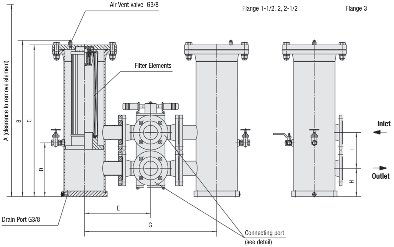
SRFL-D-160 / 200 / 300 / 600
